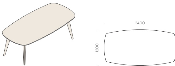
en_Meeting table with rounded top and 4 legs it_Tavolo riunioni sagomato 4 gambe fr_Table réunion avec plateau arrondi et 4 pieds
