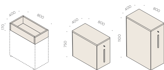
en_Planter box it_Fioriera fr_Pot à fleurs en_Low Orgatower it_Orgatower basso fr_Orgatower basse en_High Orgatower it_Orgatower alto fr_Orgatower haut
