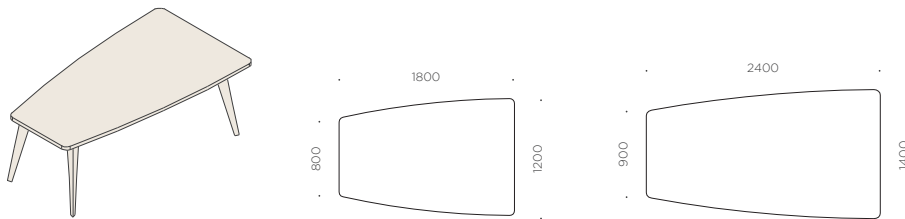
en_Meeting table with trapezoidal top and 4 legs it_Tavolo riunioni trapezoidale 4 gambe fr_Table réunion avec plateau trapézoïdale et 4 pieds
