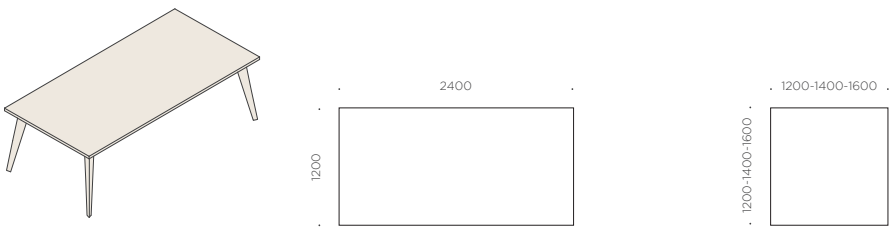
en_Meeting tables with 4 legs it_Tavolo riunioni con 4 gambe fr_Table réunion avec 4 pieds
