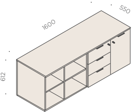
en_Structural cabinet it_Contentitore strutturale fr_Meuble porteur
