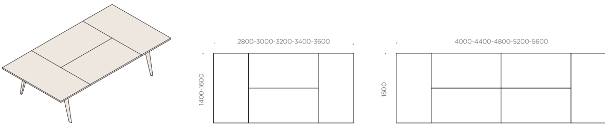
en_Meeting table with bridge leg it_Tavolo riunione gamba a ponte fr_Table de réunion avec piétements arche
