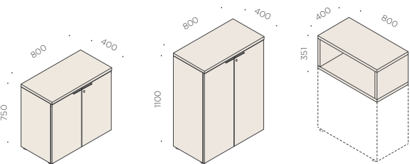
en_Side cabinet it_Contentitore laterale fr_Meuble latéral en_Side cabinet it_Contentitore laterale fr_Meuble latéral en_Open box it_Box a giorno fr_Niche ouverte
