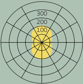
oto 01 111m/W@2700K
