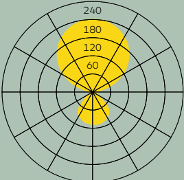
oto 34 151lm/W@4000K
