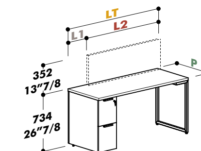
Dattilo indipendente con cass. freestanding return with pedestal/retour indépendant avec caisson/ala indipendente con buc
