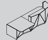
ALP22L 3034 / 1200 / 1100 119 1/2" / 47 1/4" / 43 1/4" ALP22P 3034 / 1200 / 1100 119 1/2" / 47 1/4" / 43 1/4"
