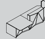
ALP22L 3034 / 1200 / 1100 119 1/2" / 47 1/4" / 43 1/4" ALP22P 3034 / 1200 / 1100 119 1/2" / 47 1/4" / 43 1/4"
