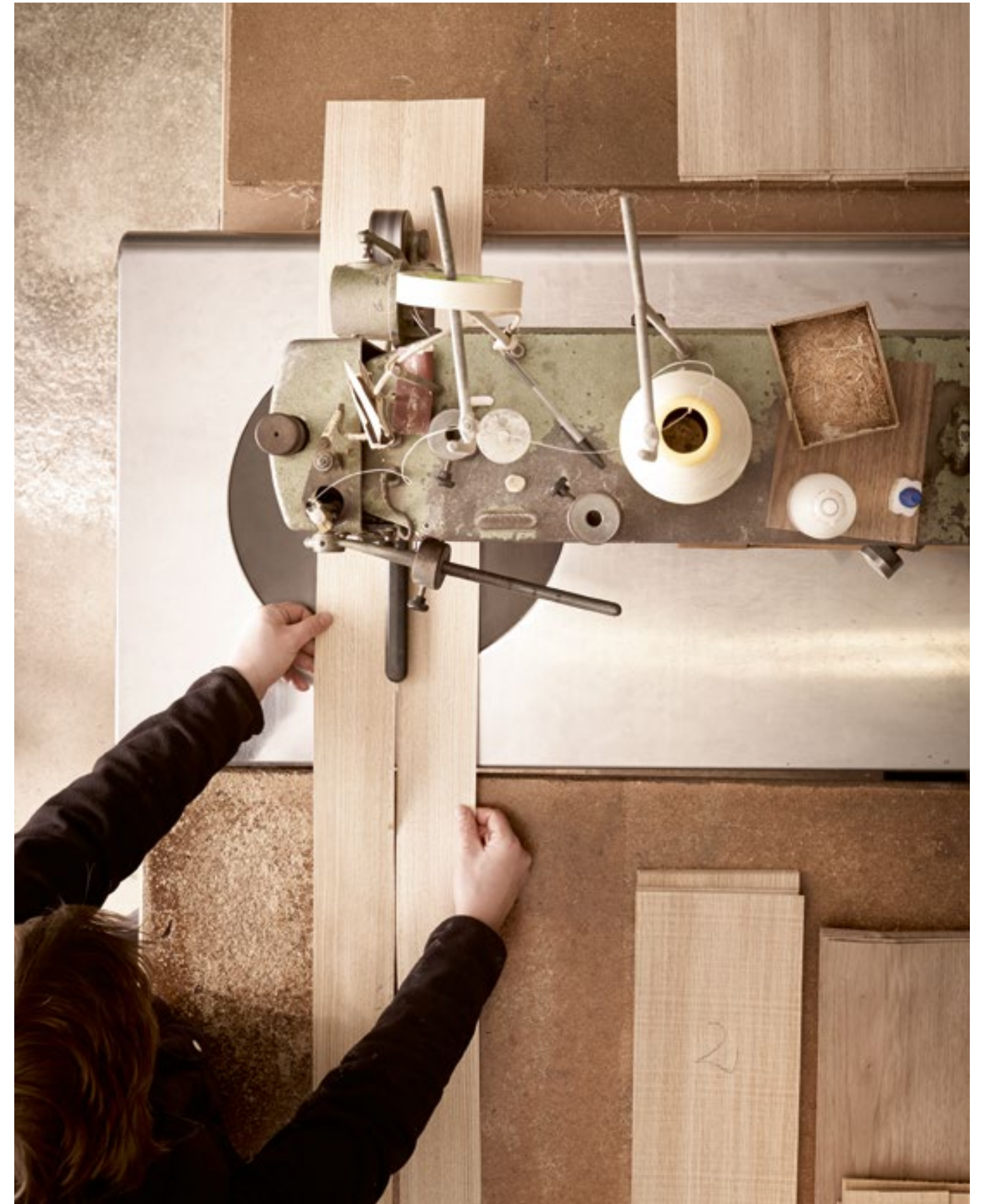
Sewing process of wood sheets. We support FSC sustainable wood sourcing Proceso de cosido de láminas de madera. Utilizamos maderas de bosques de tala controlada con sello FSC
