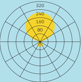
bob 30 12055lm/W@4000K
