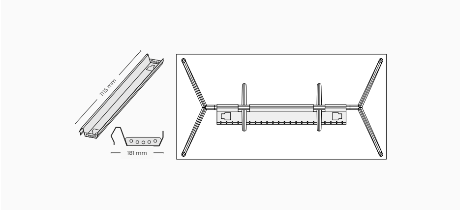
Plateau individuel en acier de 1150 mm pour tables individuelles de 1800 et 2000 mm.
