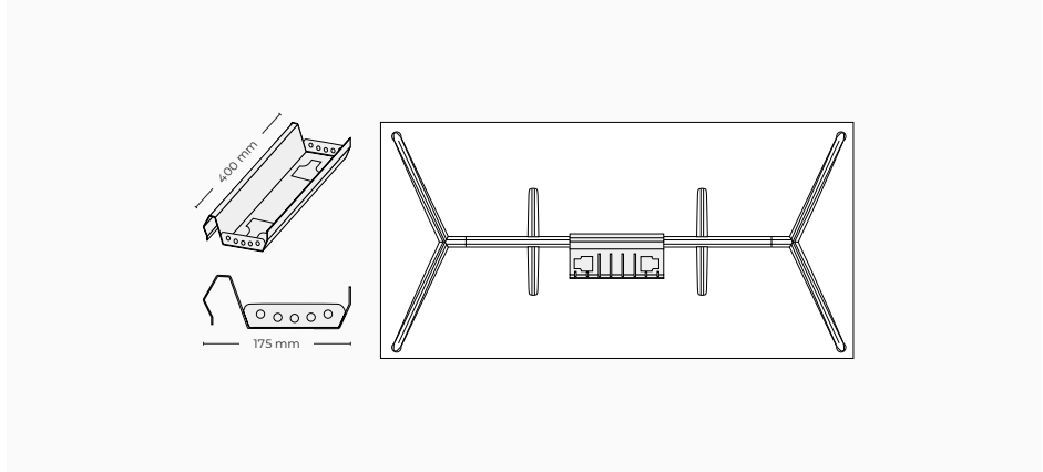
Plateau individuel en acier de 40 cm pour tables individuelles de 160, 180, 200 et 220 cm de long.
