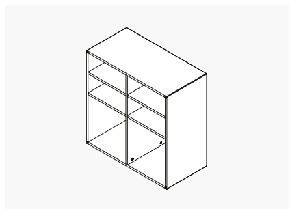
Module 7 Store W: 900 x D: 450 x H: 900 mm
