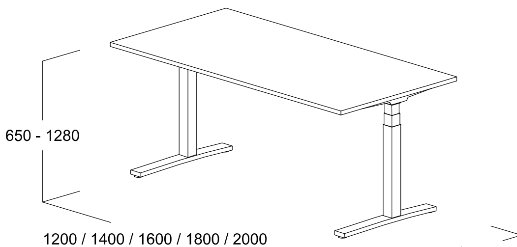
Reihe CL2 mit C-Fuß
